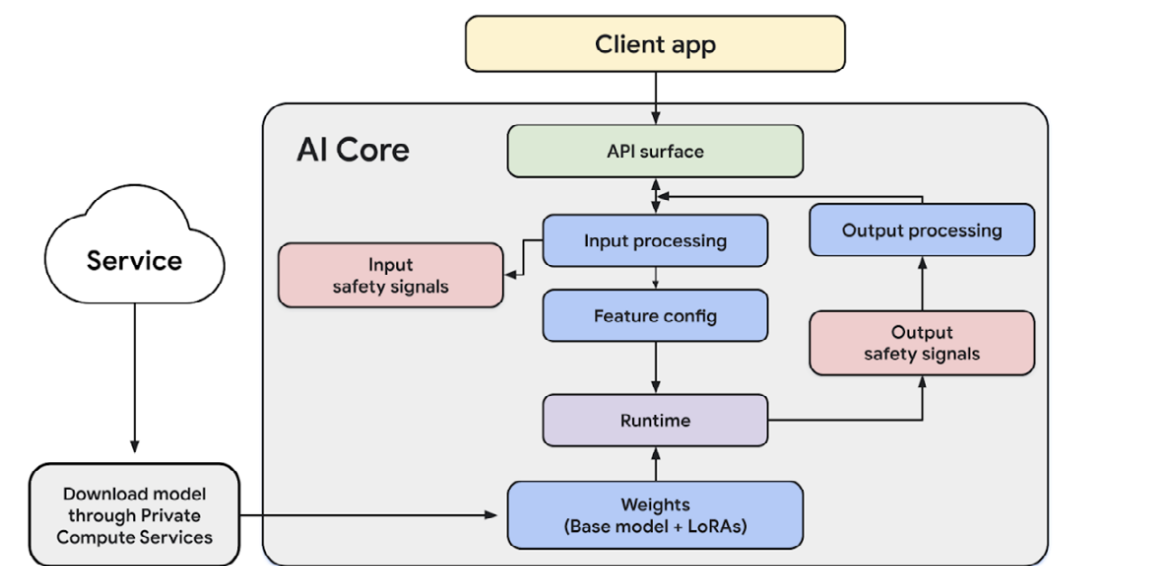
Diagrama de cómo los teléfonos Android con AI Core pueden ejecutar un modelo de lenguaje en local. Imagen: Google
