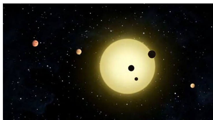
Representación artística de Kepler-11, una estrella pequeña y fría alrededor de la cual orbitan seis planetas. (foto: NASA)
