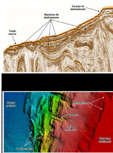
Figura 2. Ejemplo de una imagen batimétrica (abajo) y sísmica (arriba) donde se diferencian rasgos geomorfológicos correspondientes a deslizamientos submarinos. Algunos de estos eventos podrían tener la capacidad de generar tsunamis potencialmente peligrosos para las comunidades costeras.
